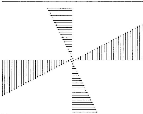
Doc. 3a. Visualisation du champ des vitesses d'un écoulement dans l'œil d'une tornade.
